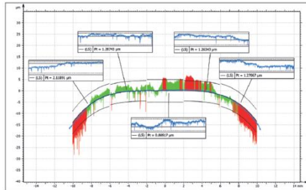
Válečkové ložisko - profil s tolerančními pásmy a chybou tvaru (Pt)
