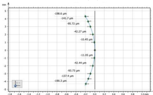
Válečkové ložisko - úbytek profilu
